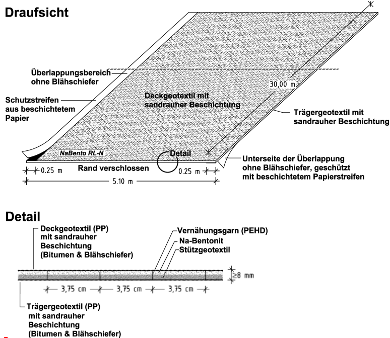
Abb. 1 Schematische Darstellung von NaBento RL-N 5000 LAGA
