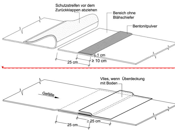
Abbildung 2 Herstellung der Überlappung
