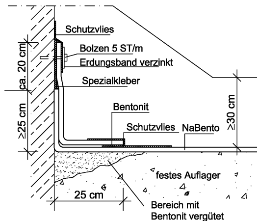
Abb. 4 Anschluss an Bauwerk
