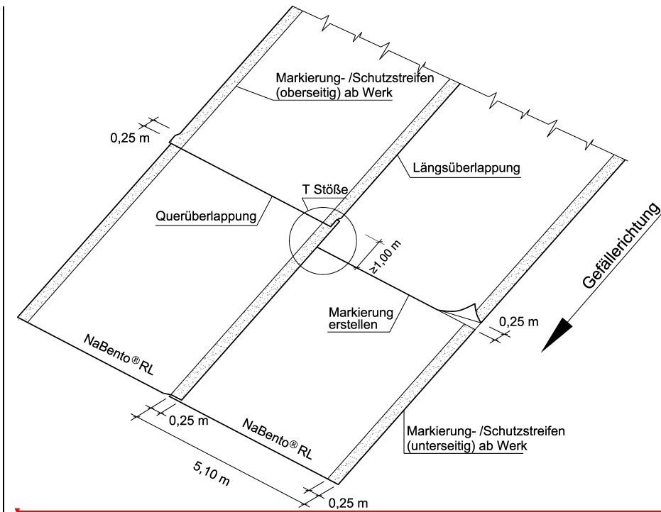
Abb. 1 Ansicht der Überlappungen/Bahnenanschlüsse von NaBento RL-N
