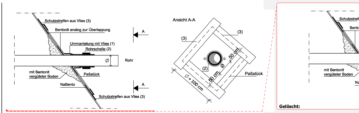
Abb. 3 Rohranschluss
