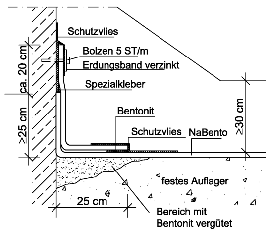
Abb. 4 Anschluss an Bauwerk
