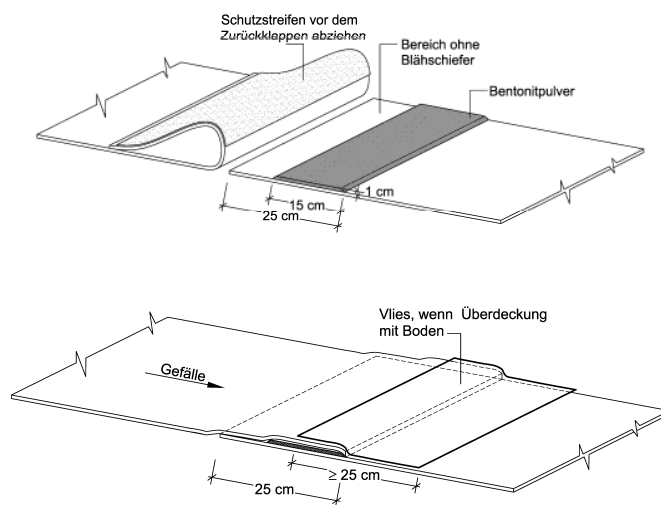
Abb. 2 Herstellung der Überlappung
