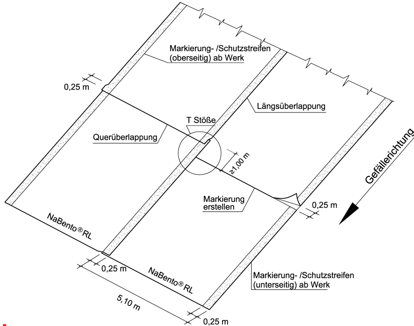
Abb. 1 Ansicht der Überlappungen/Bahnenanschlüsse von NaBento RL-C
