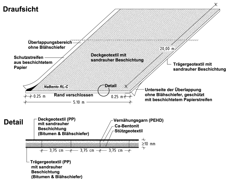
Abb. 1 Schematische Darstellung von NaBento RL-C
