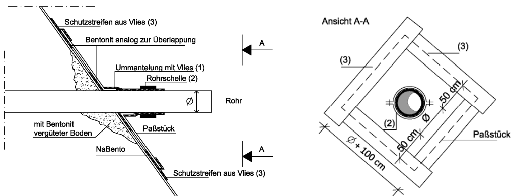
Abb. 3 Rohranschluss
